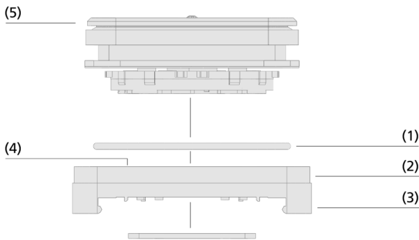
Design del sistema Adapter-Plates AP-S4
